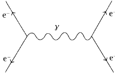
شكل خ-١: شكل فينمان الكلاسيكي لتداخلات الجسيمة.
